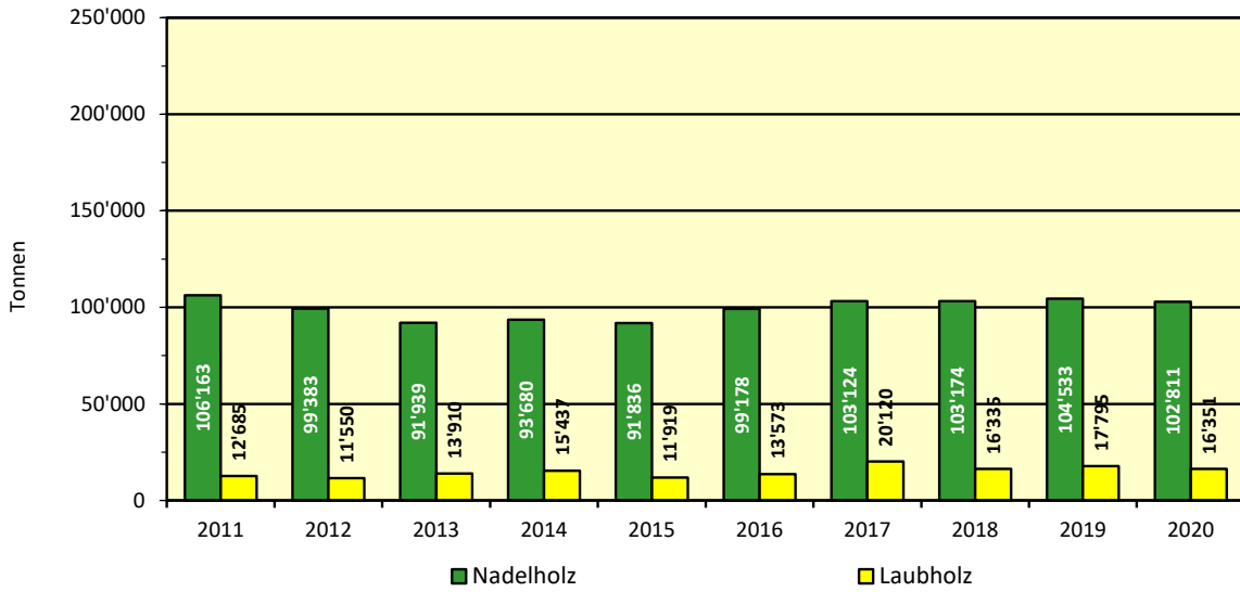
Schweizer Schnittholzexporte 2011 - 2020
