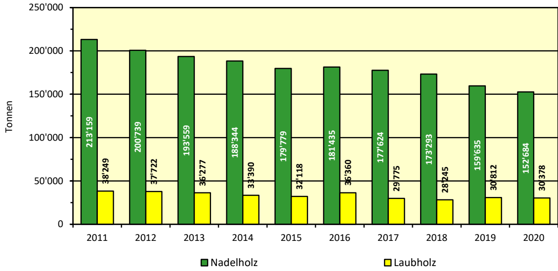
Schweizer Schnittholzimporte 2011 - 2020
